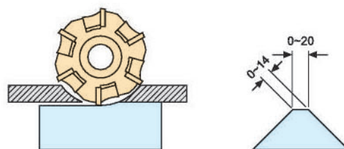
倒角圖示
